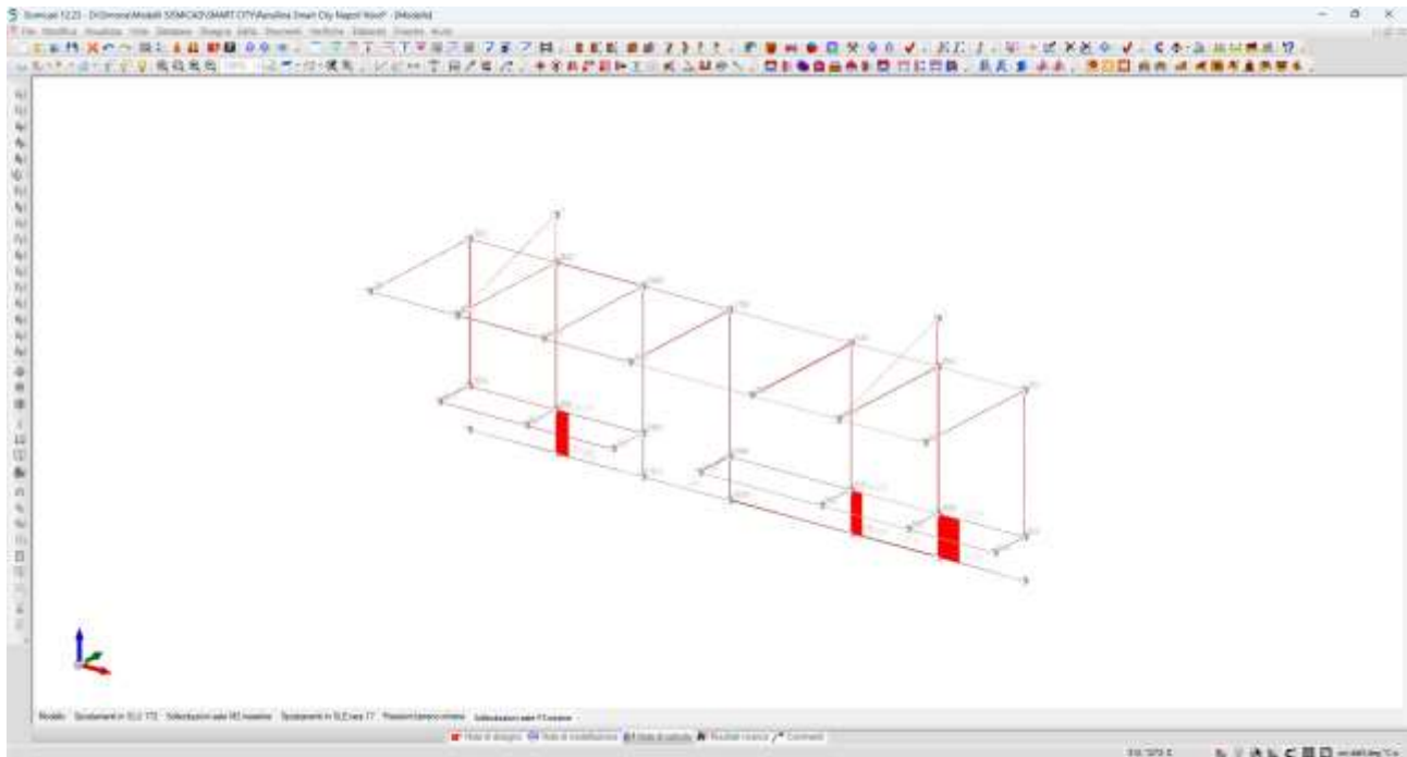
Figura 6. Involuppo taglio F3 SLU/SLV
